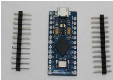
Arduino Pro Micro Atmega 32U4
