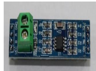
MAX485 TO TTL Module
